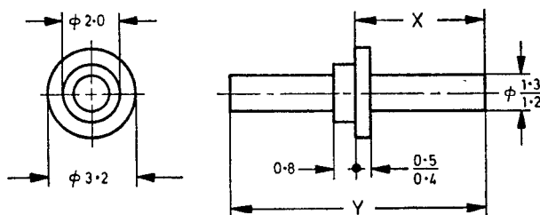
FIG. 1 TERMINAL TAG, TYPE 2
